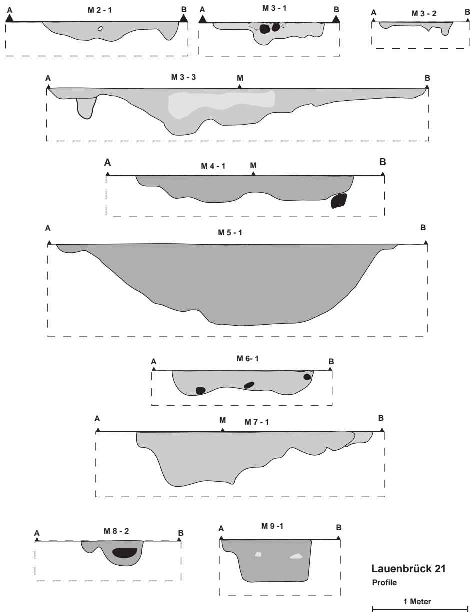
Abbildung 4: Grubenprofile Kat.Nr. 5–11, 13 und 15–16. Zeichnung: I. Neumann, St. Hesse.
